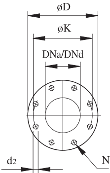
DIN 2501, Pn10/16
