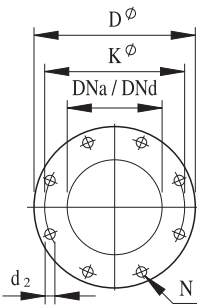
DIN 2501. Pn 10
